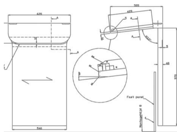
Ritningsunderlag till Kinesiska Ambassadens talarstol.
