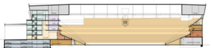
SEKTIONSSNITT AV MALMÖ ARENA.
