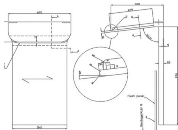
Ritningsunderlag till Kinesiska Ambassadens talarstol.
