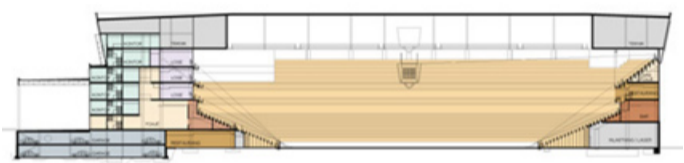
SEKTIONSSNITT AV MALMÖ ARENA.
